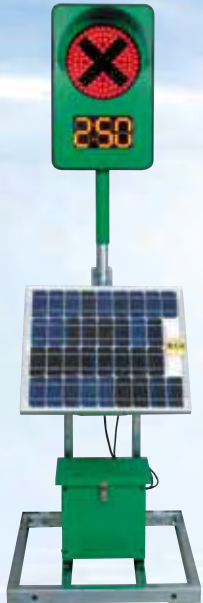
大型ソーラーパネル 大型バッテリー仕様 型式/CGS125BS-A-2
