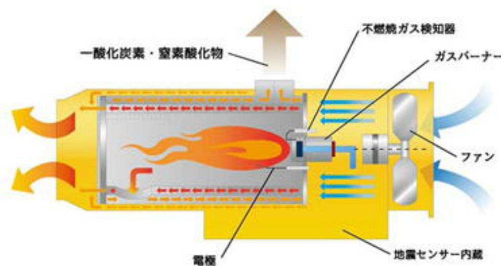
インダイレクトヒーターの仕組み
