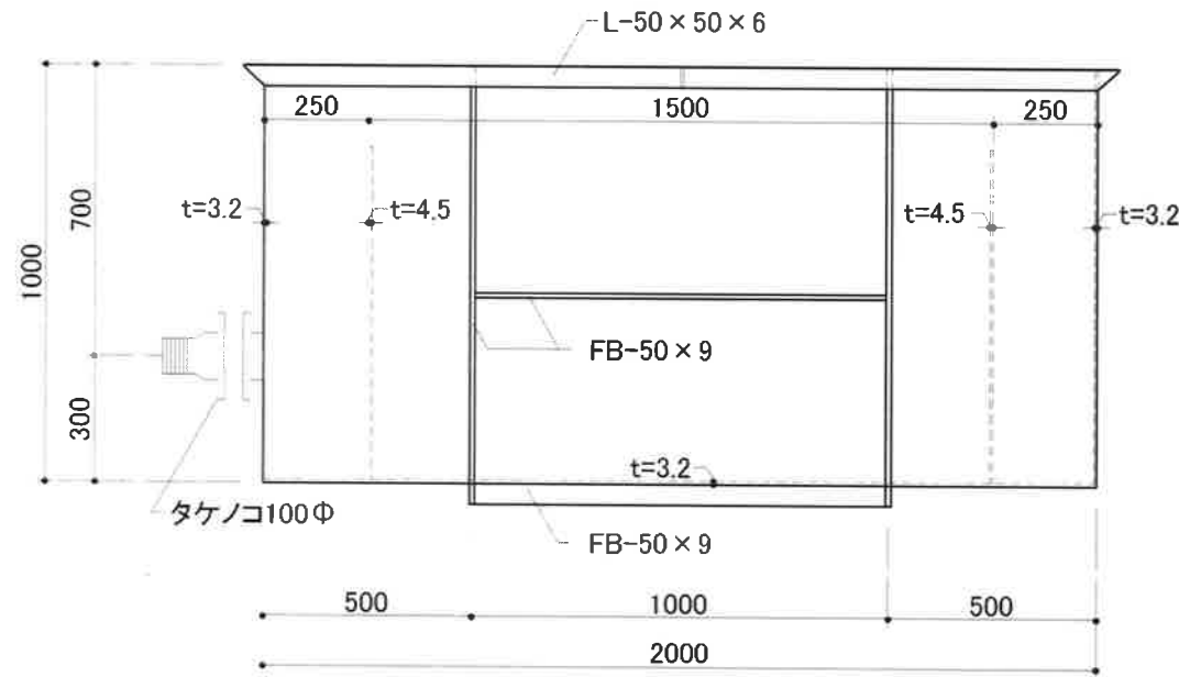
正面図
