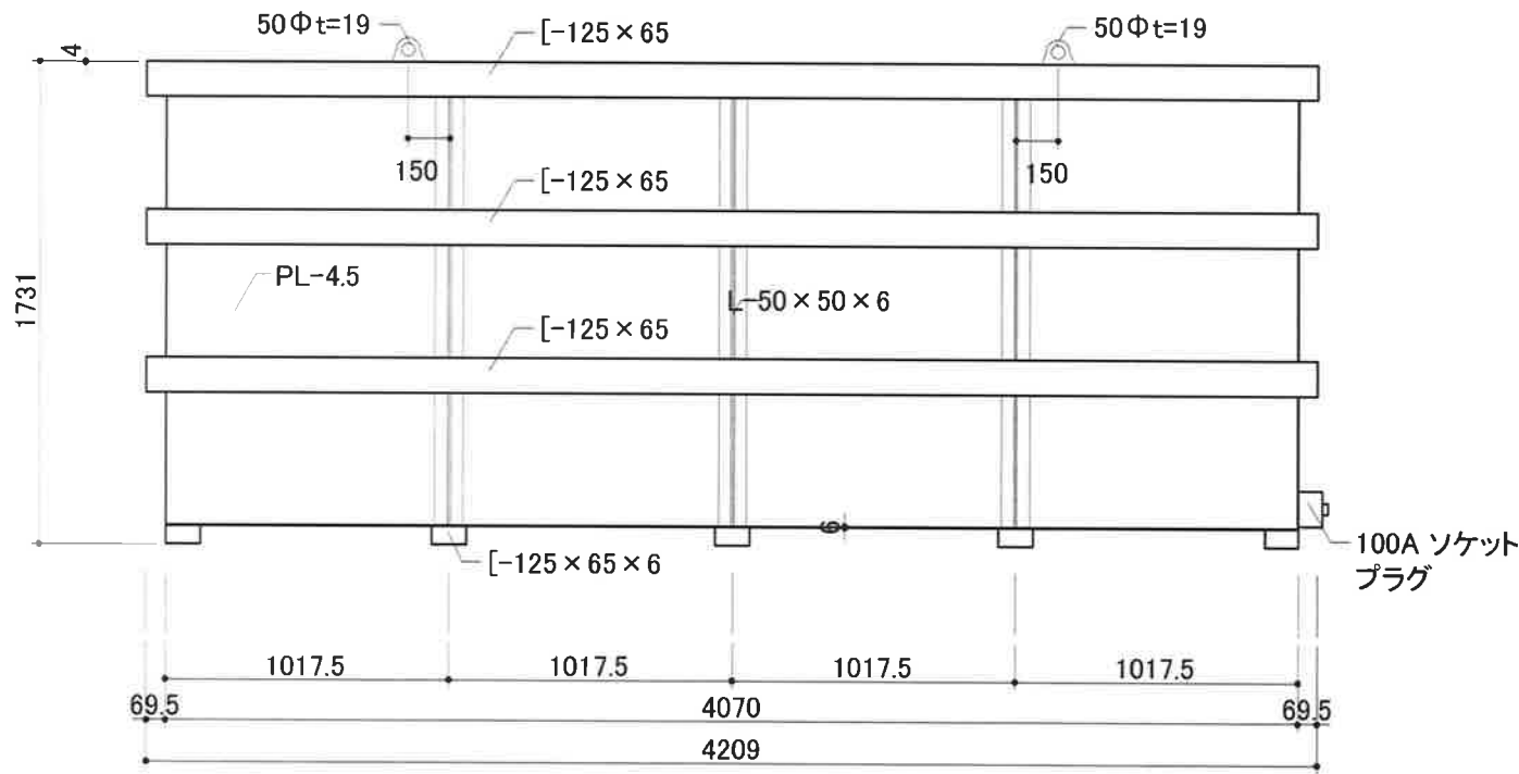
正面図
